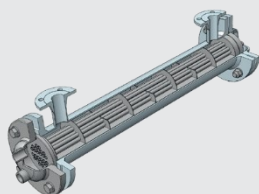
Cijevni izmjenjivač topline HCT
